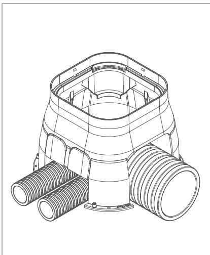
I pozzetti DrainBOX sono dotati di pretranciature per i cavidotti
