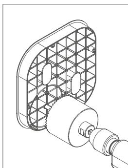
Forando il coperchio con una sega a tazza ed usando l'articolo PBR60 si possono installare pali Ø 60 mm per corpi illuminanti
