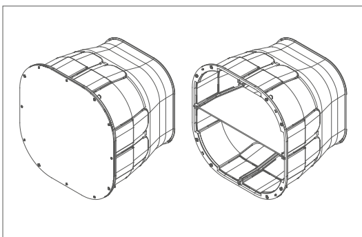
Possibilità di separare e chiudere il pozzetto sul fondo
